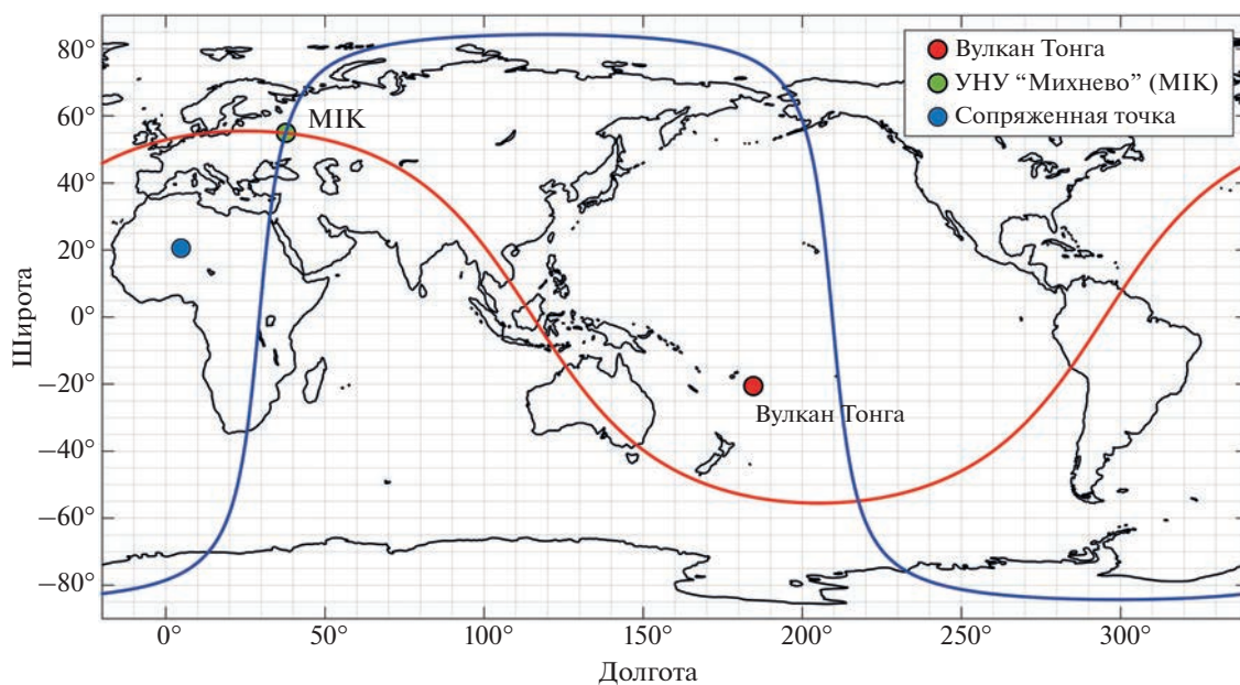
Рис. 5. Дуги большого круга, проходящие через оси магнитометров каналов H_x и H_y обсерватории МИК.
