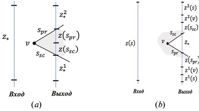
Рис. 6. Изменение Статуса при событиях "Левая вершина": (a) выпуклая, (b) вогнутая.
