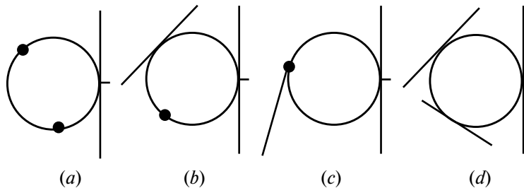
Рис. 11. Вычисление касательного круга для двух сайтов и заматающей прямой: (a) – сайты-точки, (b, c) – сайт-точка и сайт-сегмент, (d) – два сайта-сегмента.
