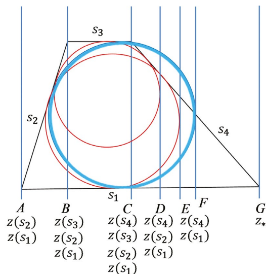
Рис. 9. Заметание четырехугольника, события вершины — A, B, C, G , события-круги D, E, F , изменения Статуса по событиям.
