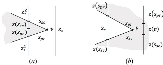
Рис. 8. Изменение Статуса при событиях “Правая вершина”: (a) выпуклая, (b) вогнутая.
