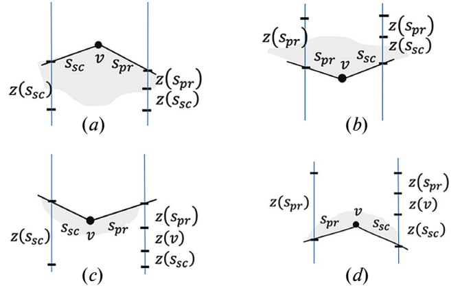
Рис. 7. Изменение Статуса при событиях "Проходная вершина": (a) верхняя выпуклая, (b) нижняя выпуклая, (c) верхняя вогнутая, (d) нижняя вогнутая.
