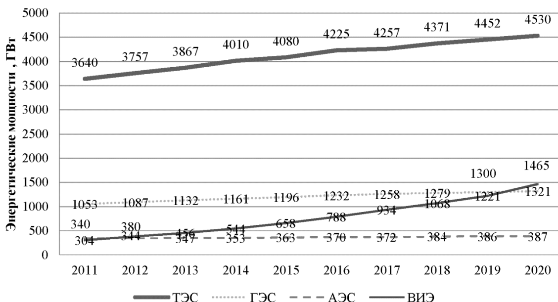
График 2. Мировые энергетические мощности за 2011–2020 гг. (ГВт). Graph 2. World energy capacity for 2011–2020 (GW).
