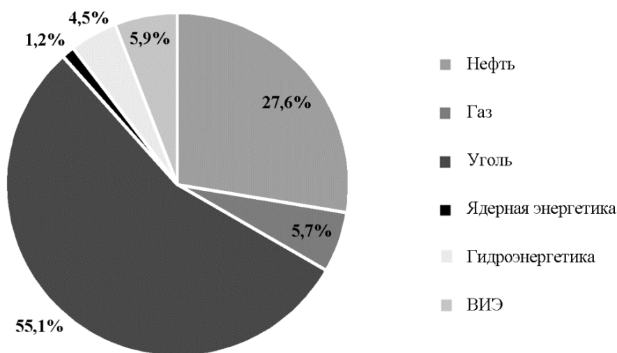
Диаграмма 1. Первичное энергопотребление Индии, 2022.
