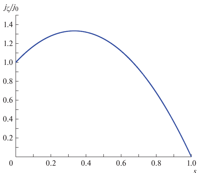
Рис. 2. Плотность тока, предписанная формулой (18) с k = 1 .
