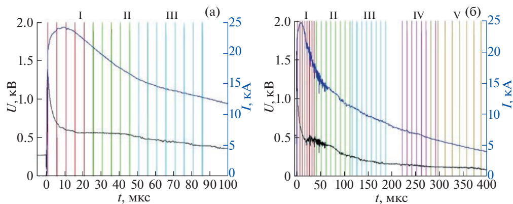
Рис. 7. Осциллограммы напряжения и тока для режимов разряда, показанных на рис. 8 и 9. Вертикальные линии показывают моменты времени на горизонтальной оси, в которые были сняты соответствующие изображения на рис. 8 и 9. а) азот, P = 4 Торр; б) P = 50 Торр. h = 30 мм, U_0 = 5 кВ.
