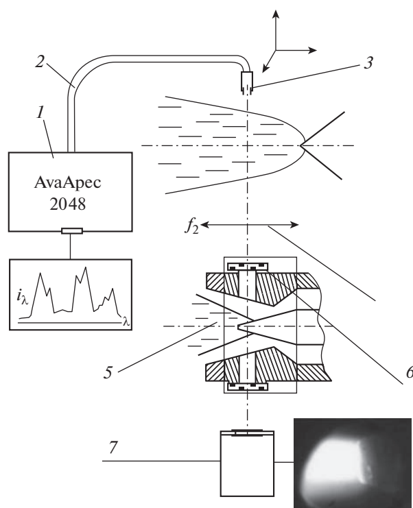
Рис. 1. Схематический чертеж ГНП с системой оптических измерений: 1 – спектрограф AvaSpec 2048 или ДФС-452 с матрицей Andor, 2 – оптоволоконно, 3 – система крепления и перемещения оптоволокон, 4 – фокусирующая линза, 5 – дуга, 6 – кварцевые окна, 7 – высокоскоростная камера типа Phantom Miro M110 с объективом “Гелиос 40-2”.
