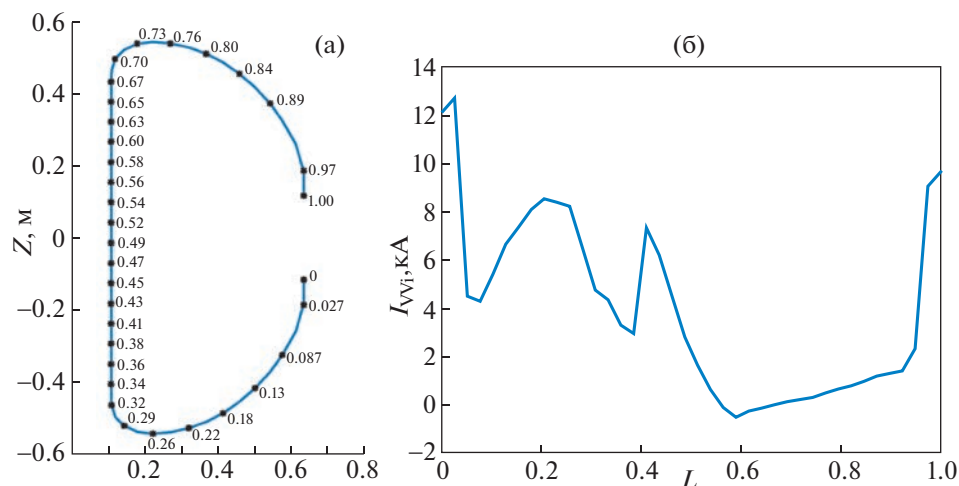
Рис. 14. а) — сечение вакуумной камеры с указанием отсчета полоидальной длины в относительных единицах (текущая длина l , разделенная на полную длину периметра за вычетом патрубков диаметром 400 мм во внешнем кольце); б) — распределение наведенного тороидального тока камеры I_{VI} по полоидальной длине в разряде 42 145 в момент времени t \approx 202.3 мс (максимальный ток при срыве I_{VI} \approx 160 кА).
