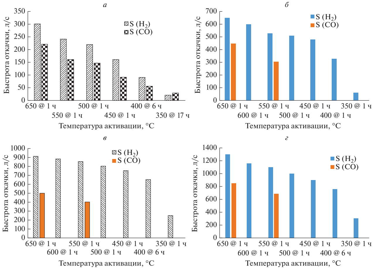
Рис. 4. Скорость откачки геттерных насосов по водороду и СО при различных температурах активации.
