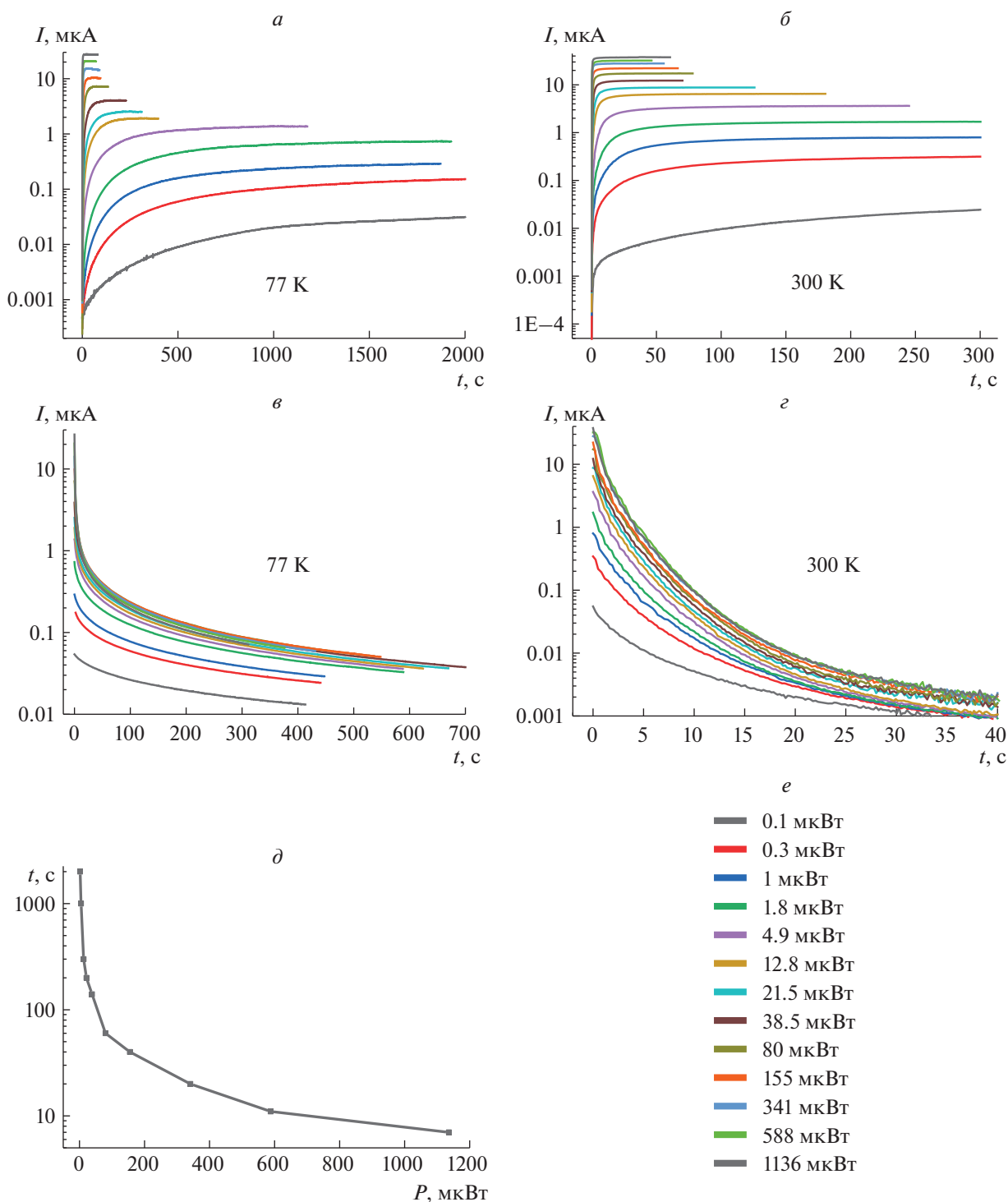
Рис. 3. Зависимости роста (а, б) и релаксации (в, г) фототока в образце ZnSe:Fe 1.5% при облучении его излучением с длиной волны 505 нм при различных температурах и мощности излучения (е), а также зависимость времени выхода фототока на насыщение от мощности излучения (д).
