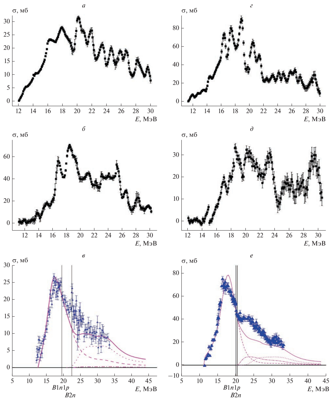
Рис. 1. Сравнение (для ^{58}\text{Ni} слева, для ^{60}\text{Ni} справа) сечений фотонейтронных и фотопротонных реакций, полученных в разных экспериментах, с результатами расчетов в КМФЯР: а и г – (\gamma, sn) [4], б и д – (\gamma, p) [5], в и е – (\gamma, xn) [6] (треугольники) и сечения реакций на ядре ^{58}\text{Ni} , рассчитанные теоретически [7] ( \sigma^{\text{теор}}(\gamma, xn) – сплошная линия; \sigma^{\text{теор}}(\gamma, 1n) – пунктирная линия; \sigma^{\text{теор}}(\gamma, 1n1p) – точечная линия; \sigma^{\text{теор}}(\gamma, 2n) – штрих-пунктирная линия).
