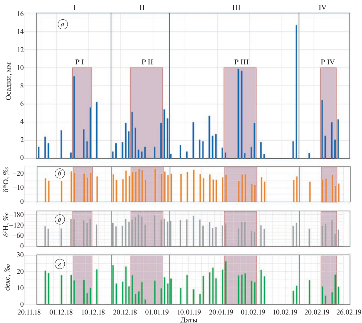
Рис. 3. Вариации значений: количества осадков ( a ), \delta^{18}\text{O} ( б ), \delta^2\text{H} ( в ), d_{\text{ex}} в осадках (снеге) ( г ), отобранных на метеороbservатории МГУ в день их выпадения, в чёрные рамки заключены осадки, в результате аккумуляции, которых сформировалась слой I, II, III и IV; тёмным фоном выделены осадки, в результате аккумуляции которых сформировалась часть слоя (проба), отобранная для определения \delta^{18}\text{O} (см. рис. 4).
