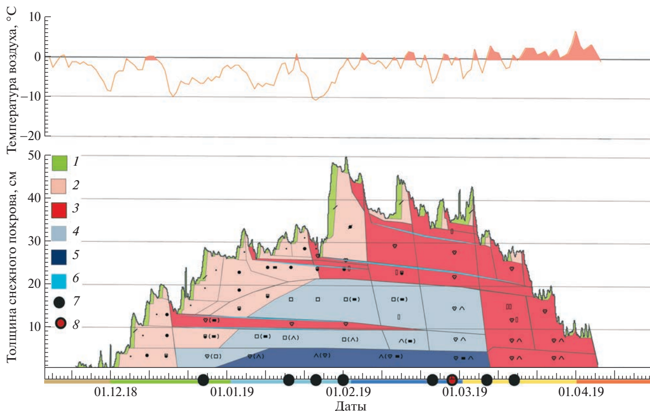
Рис. 1. Схема изменения строения снежной толщи в Москве зимой 2018/19 г. и температура воздуха по данным измерений на метеорологической обсерватории МГУ (Москва): 1 – свежеснежавший снег; 2 – мелкозернистый и среднезернистый осевший; 3 – таяния–замерзания; 4 – с огранкой; 5 – глубинная изморозь; 6 – лёд; 7 – даты измерений в шурфах и траншеях; 8 – даты отбора проб в траншее. Условные и цветовые обозначения соответствуют (Фирц и др., 2012).
