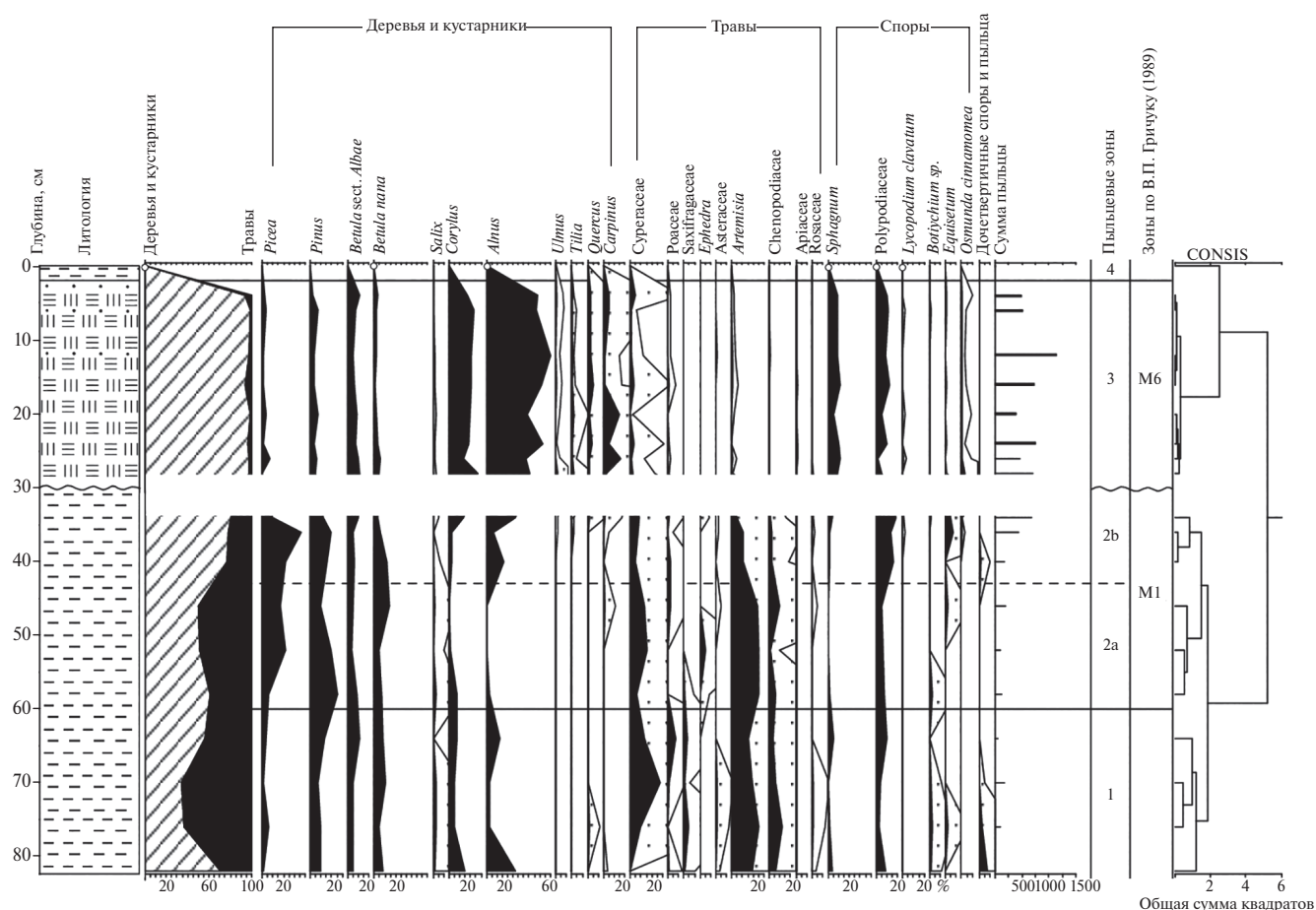
Рис. 8. Спорно-пыльцевая диаграмма отложений разреза "Граничная".
