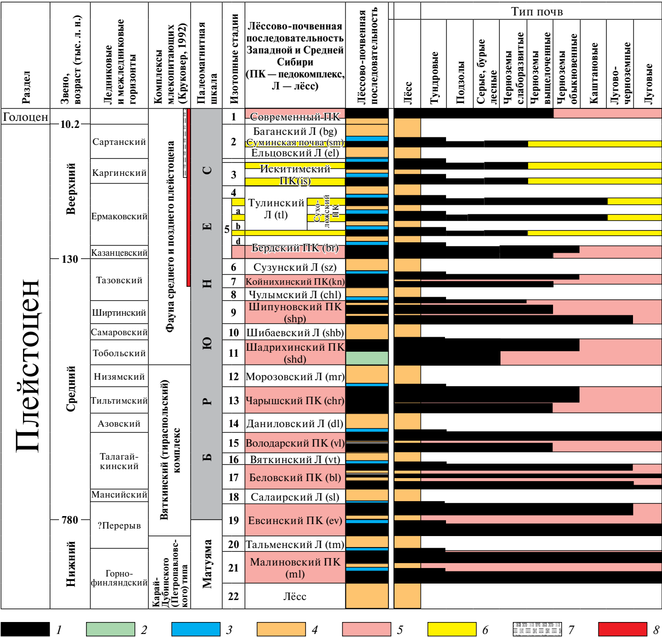
Рис. 1. Стратиграфическая схема лёссово-почвенной последовательности плейстоцена Сибири (Зыкина, Зыкин, 2012, с уточнениями). Горизонты почв: 1 — гумусовые, 2 — иллювиальные; 3 — криогенные образования; 4 — лёссы; 5 — стадии потепления; 6 — холоднее и короче, чем голоцен; интервалы: 7 — имеющие 14 C-даты, 8 — имеющие люминесцентные даты; ПК — педокомплекс; Л — лёсс. Fig. 1. Stratigraphic scheme of the loess-soil sequence of the Pleistocene of Siberia (Zykina, Zykin, 2012, with refinement). Soil horizons: 1 — humus soil horizons, 2 — illuvial soil horizons; 3 — cryogenic formations; 4 — loess; 5 — stage warming; 6 — colder and shorter than the Holocene; intervals: 7 — interval having 14 C date, 8 — interval having luminescent dates; ПК — pedocomplex; Л — loess.
