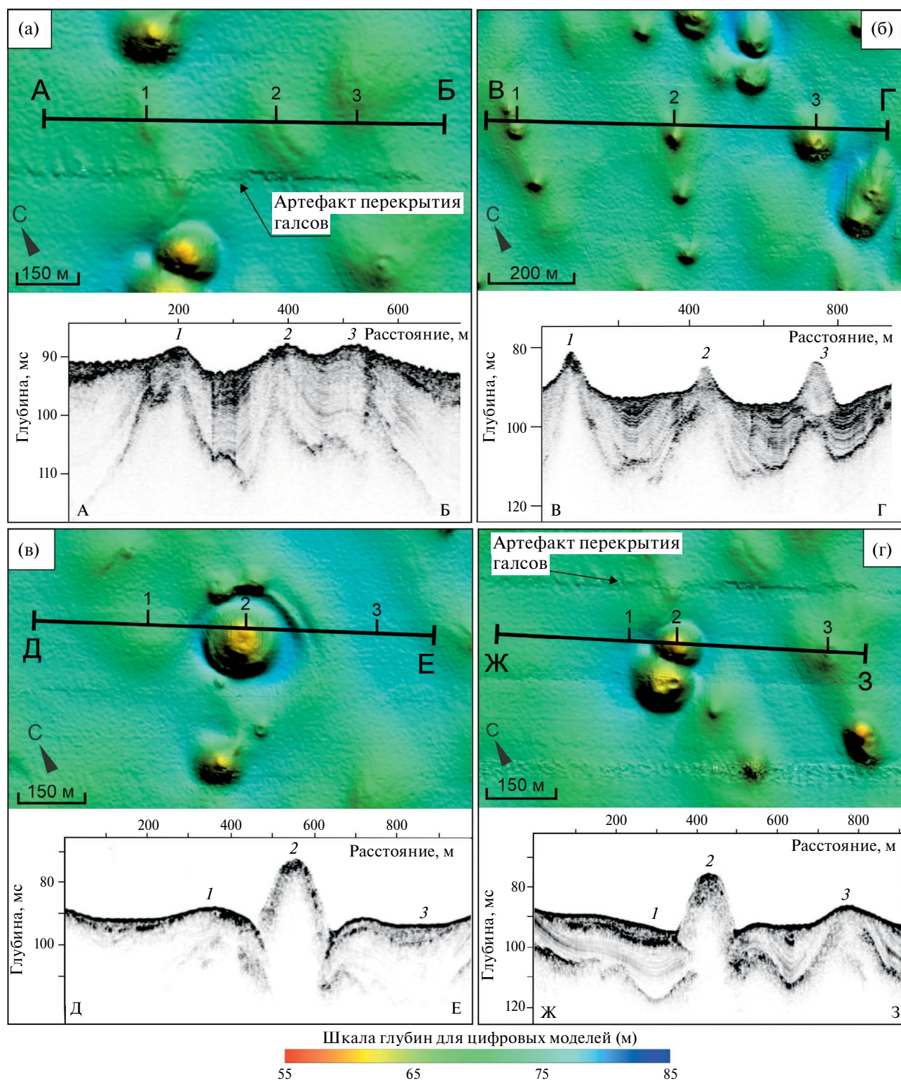
Рис. 4. Морфология и внутреннее строение валов (а), впадин (б) и пингоподобных форм (в, г) (местоположение участков показано на рис. 2, (а)). Для каждого участка приведен фрагмент ЦМР и соответствующий профиль, полученный методом высокочастотного сейсмического профилирования. Цифрами на профилях (т. 1–3) показаны формы рельефа (впадины, валы, ППФ), упоминаемые в тексте.
